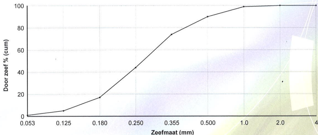
Korrelverdelingsdiagram
