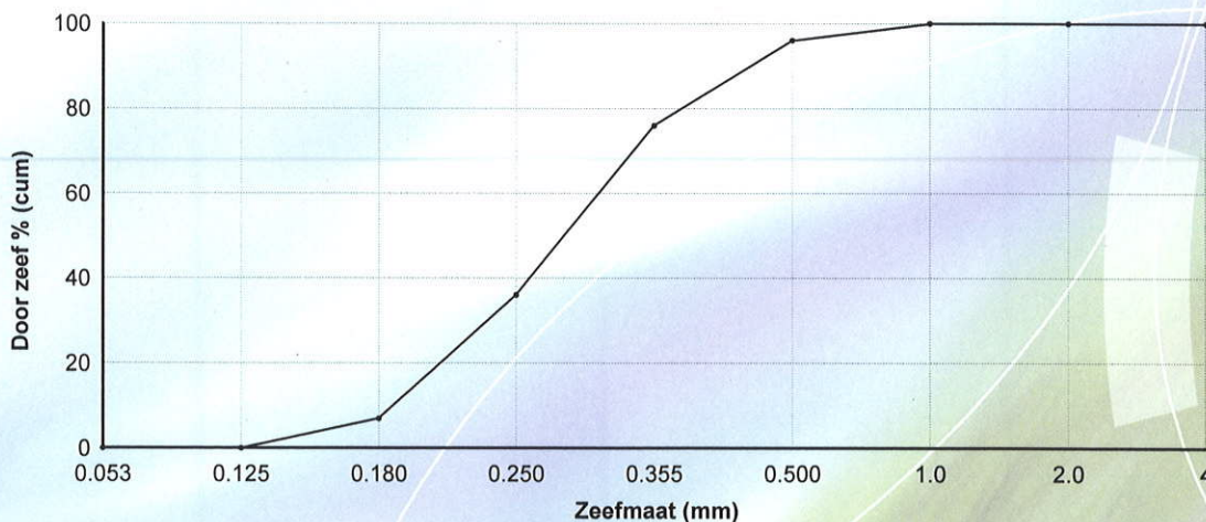
Korrelverdelingsdiagram
